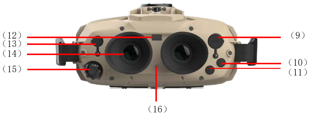
图 3 手持后部
